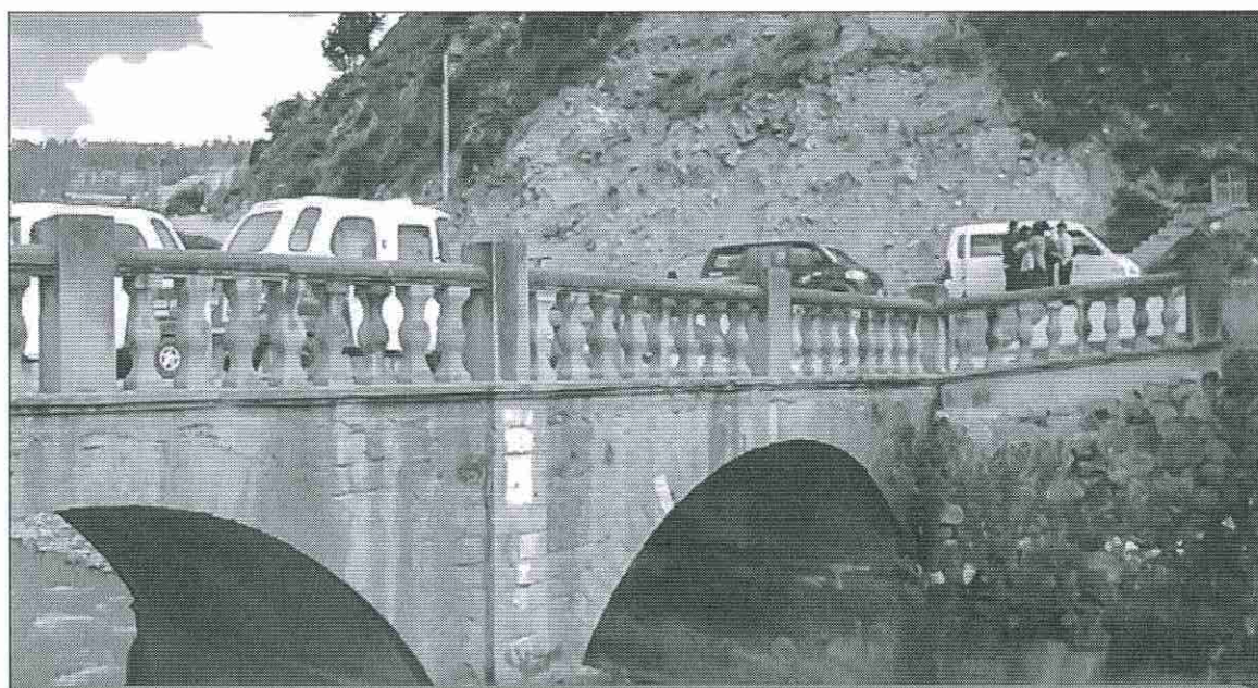
Fotografías 11 y 12: Puente Colonial de Chumbao: Fue construido a base de cal y piedra en el periodo de la colonia y en la actualidad da acceso a los poblados de que se ubican en la margen derecha del río. Construido en 1776 bajo el mando del corregidor Jacinto Camargo en el periodo del Virrey Amat. Medidas del puente Chumbao; Longitud 17 metros y un ancho de 4 metros aprox. Situado sobre el río que le da su nombre, ubicado bajo las faldas del mirador natural del cerro Huayhuaca.
