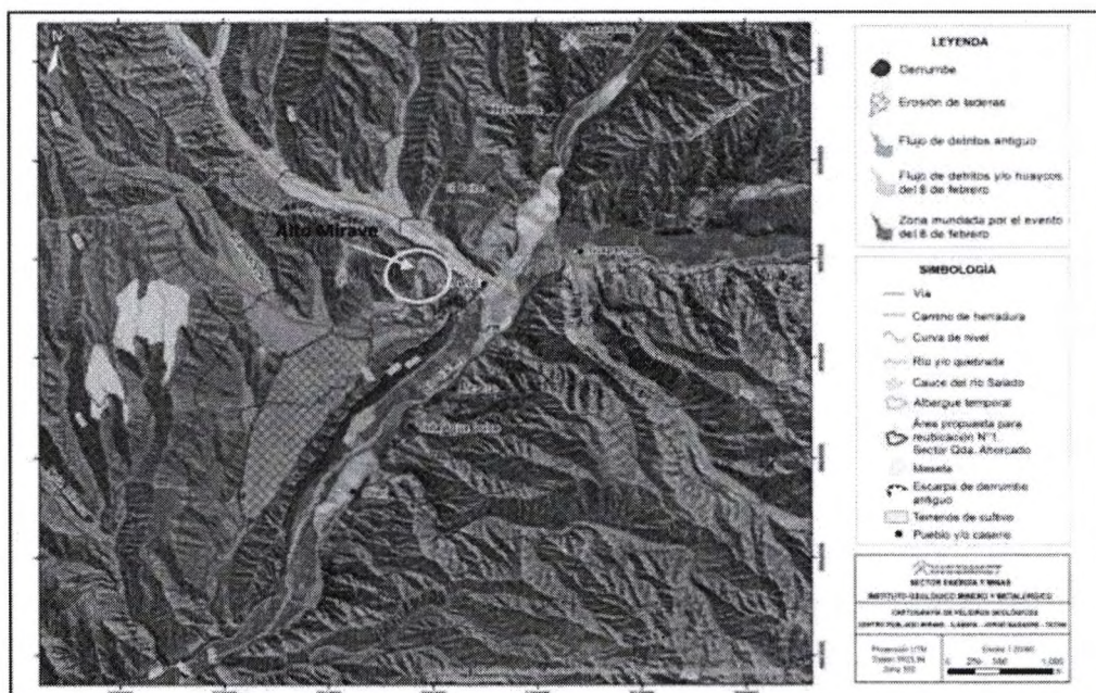
Mapa de peligros geológicos de los sectores de Mirave y Quebrada Ahorcado. Informe técnico N° A6896, según Opinión Técnica N° 007-2020
