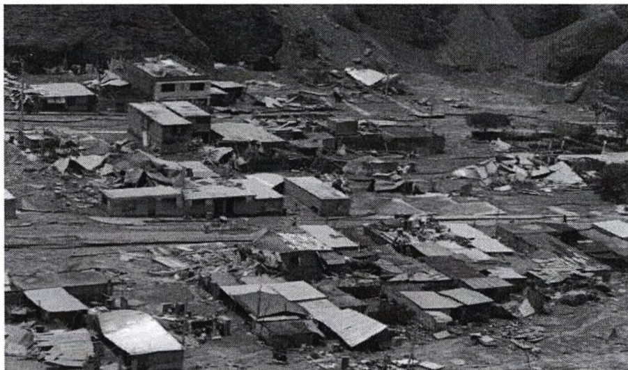
Efectos del Huayco del 8 de febrero del 2019 en Mirave.
