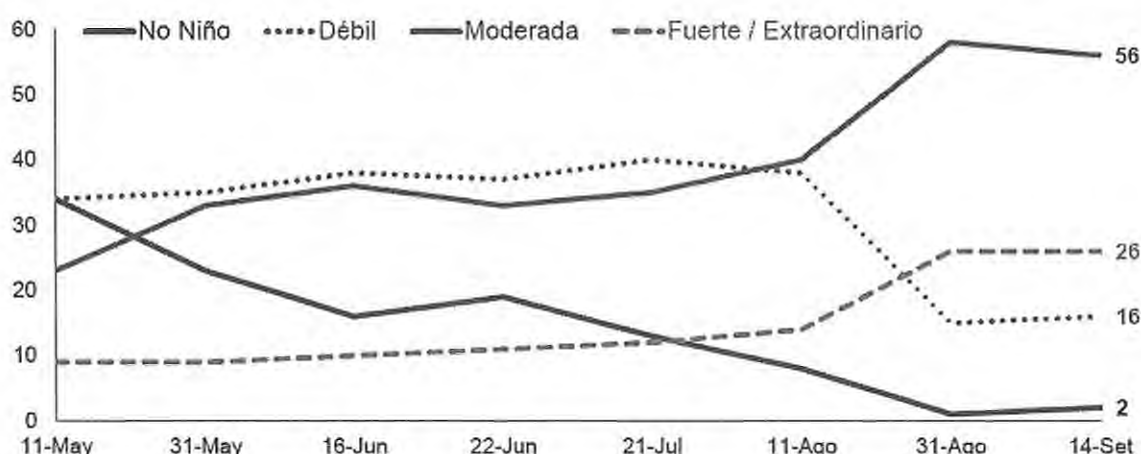
Probabilidad de ocurrencia de el niño costero en Perú para el verano 2024 (%)
