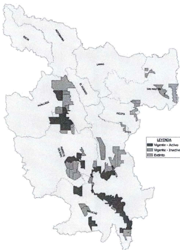
Figura 2. Concesiones forestales con fines maderables en la región San Martín
