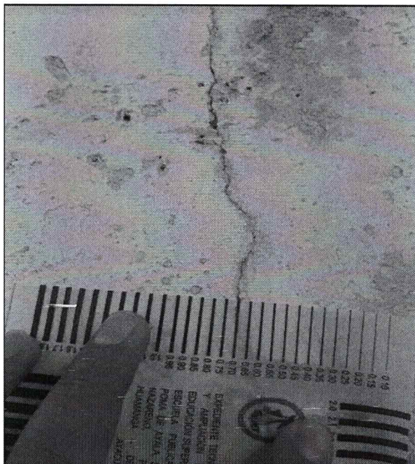
Fotografía 5. Rajadura en pared de 2cm.
