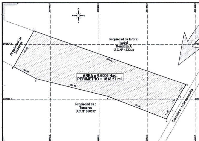
IMAGEN N° 01 PLANO PERIMÉTRICO DEL TERRENO DESTINADO PARA LA CONSTRUCCIÓN DE LA UNAMAZ
