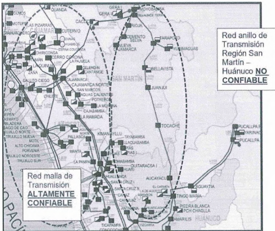
Plano del Sistema de Transmisión marzo 2024 Fuente: COES
