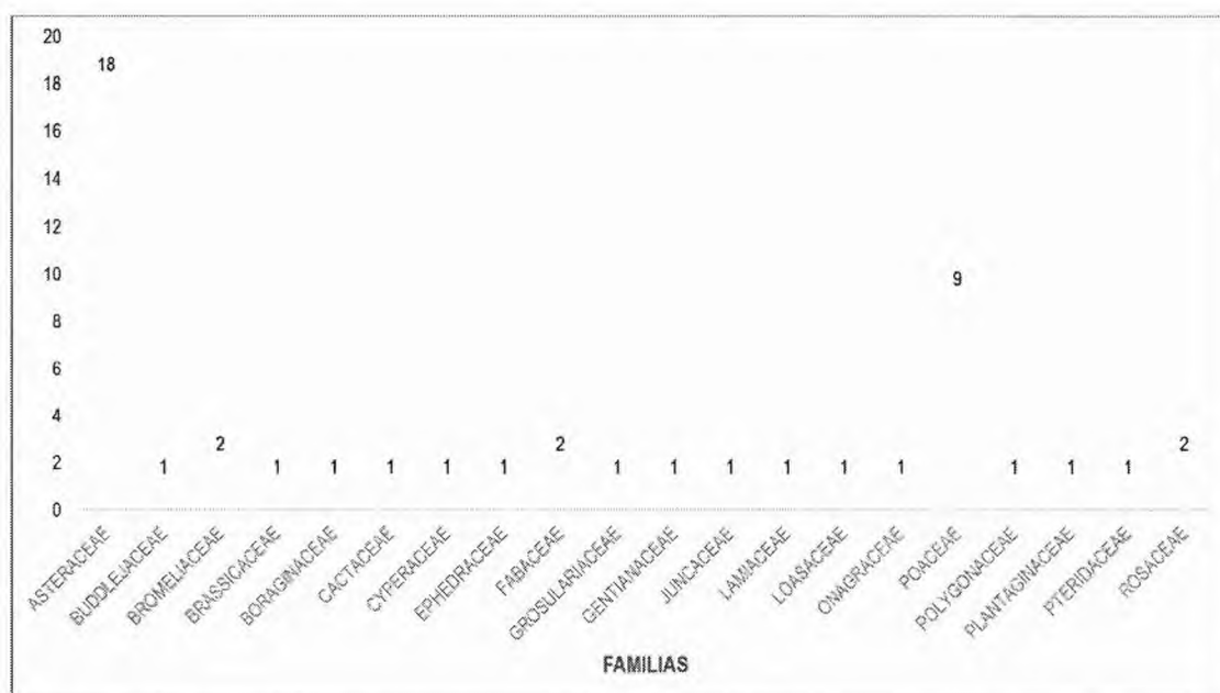
Figura 3. Especies de cada familia, en ecosistemas de ph-SaS.
