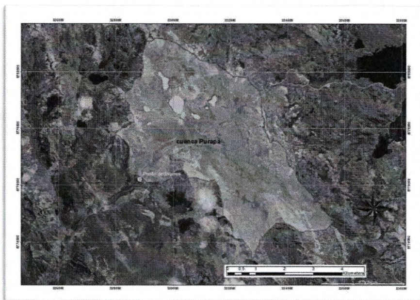
Figura 02: Mapa satelital de la cuenca Purapa y red de drenaje
