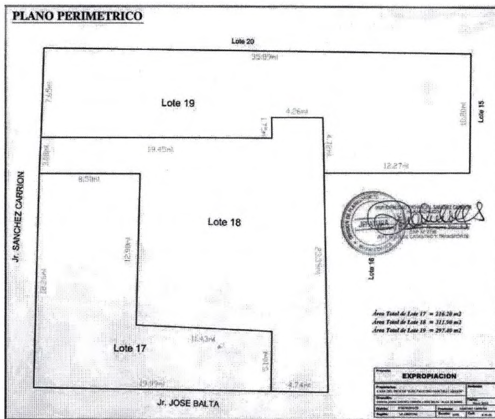
Gráfico N° 02 Plano perimétrico de la Casa del Prócer Faustino Sánchez Carrión
