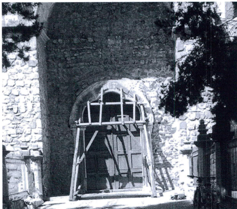
ESTRUCTURAS DÉBILES
