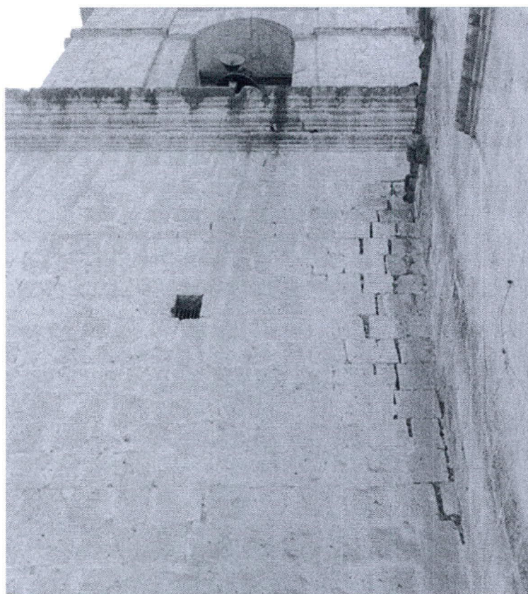
PAREDES RESQUEBRAJADAS
